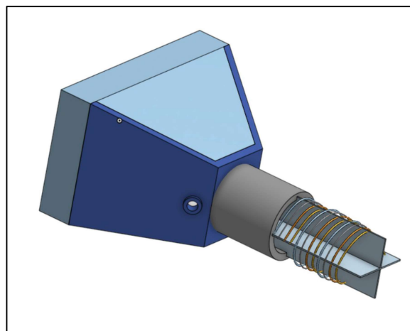
Lilitan Elemen Pemanas
