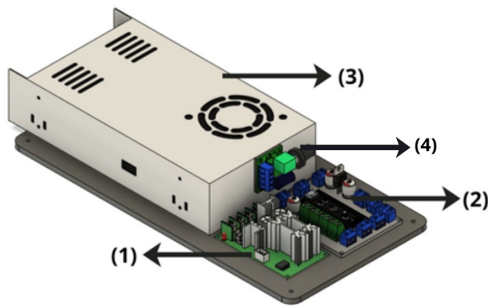
Bagian Dalam Modul Pemanas Udara
